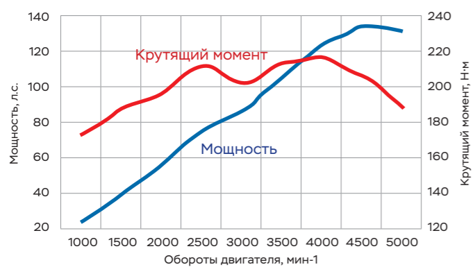
ВНЕШНЯЯ СКОРОСТНАЯ ХАРАКТЕРИСТИКА
